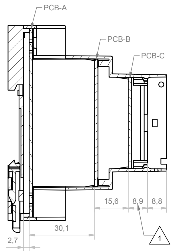
A-A (1:1)
